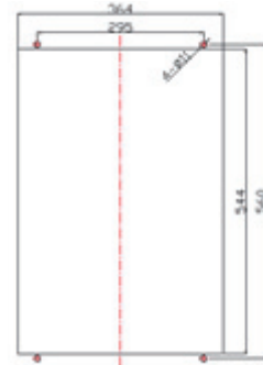
穿墙安装开孔尺寸
