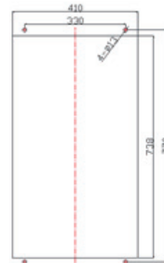
穿墙安装开孔尺寸
