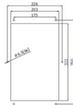
穿墙安装开孔尺寸
